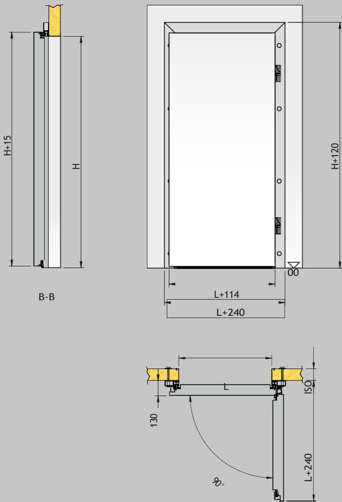
Fissaggio su pannello *
