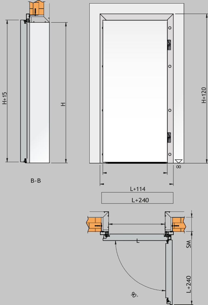
Fissaggio su muratura con imbotte *
