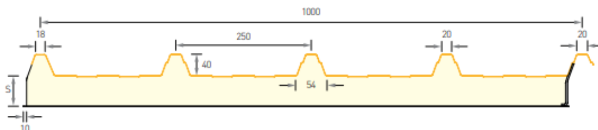
DISEGNO TECNICO AGROPANEL
